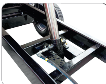
Pneu do Rodado: 7.50 x 16 CBFA 6: 2 eixos com rodado duplo no eixo traseiro
