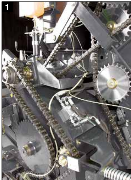
Transmissão simples, embreagem do came protegida
