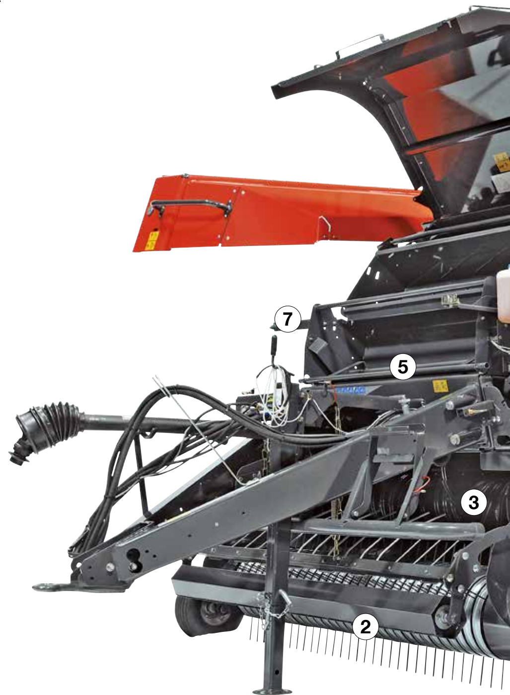
Transmissão simples, embreagem do came protegida
